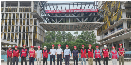
钢结构连廊整体提升效果
