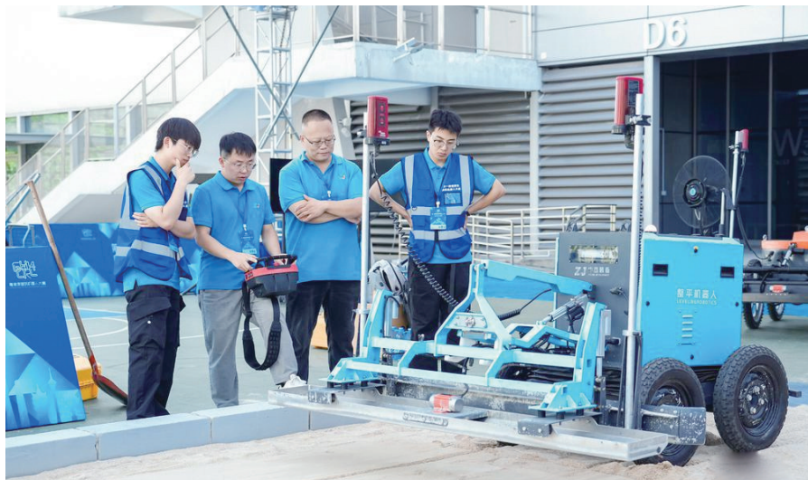
第一届粤港澳建筑机器人大赛竞赛现场——地面整平机器人作业中（图源：广东省住房和城乡建设厅）
