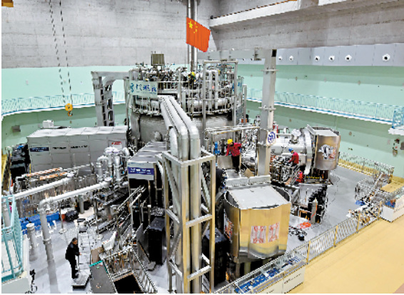
■全超导托卡马克核聚变实验装置(EAST)。
