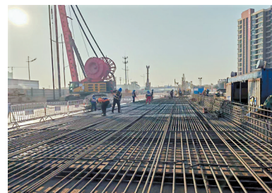
■江府站地连墙钢筋施工。 广州地铁供图
