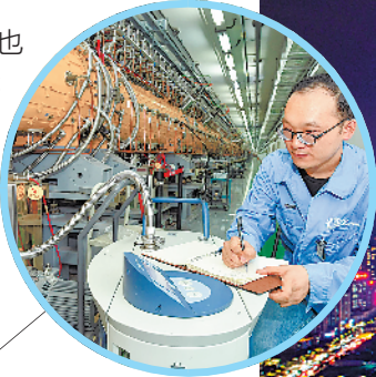
工程师在东莞中国散裂中子源检查直线加速器工作情况
