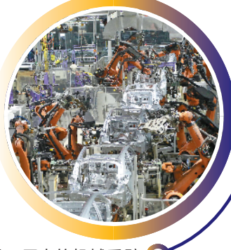
增城工厂内的机械手臂 宋韵潇 摄
