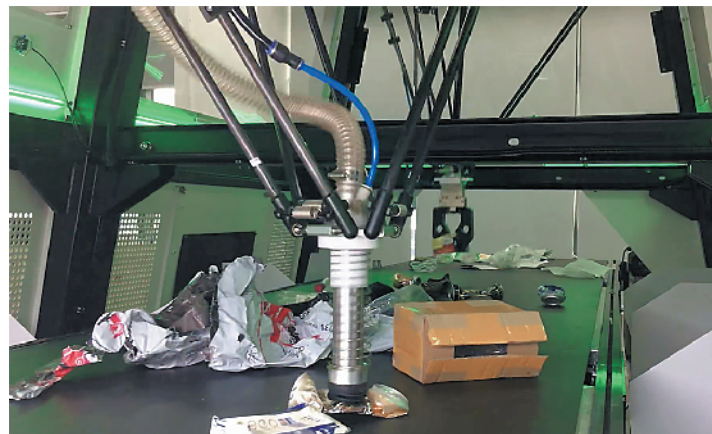
生活垃圾分拣机器人可识别数十种可回收物品(弓叶科技供图)
