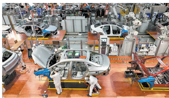
广汽埃安番禺总装车间
