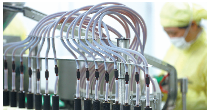
口服液生产线罐装设备
