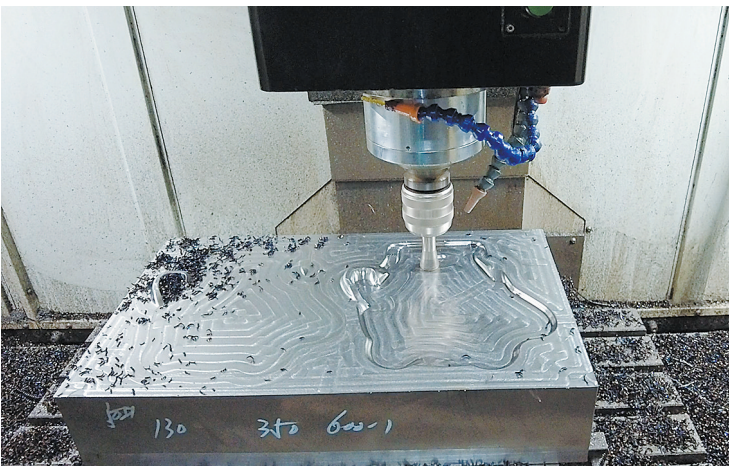
东莞一企业正在赶制一批“冰墩墩”外壳模具
