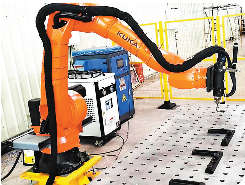
大捷智能复杂曲面、高精度机器人抛光打磨与感应淬火装备 受访方供图
