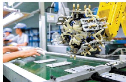
广东省东莞市松山湖长盈精密技术有限公司的智能手机部件生产线
