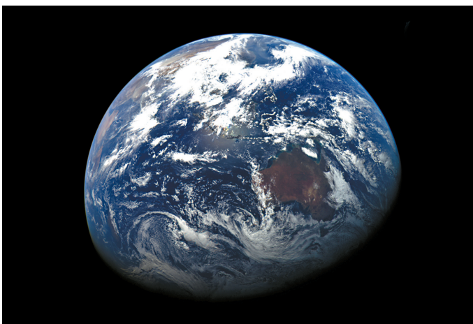
■天问二号探测器拍摄的地球彩色图。 新华社发
