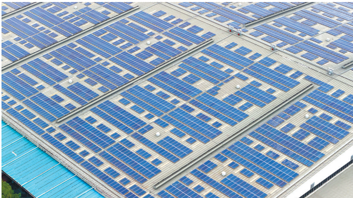
珠海科技产业集团位于顺德北滘镇的5.5兆瓦 分布式光伏发电项目
